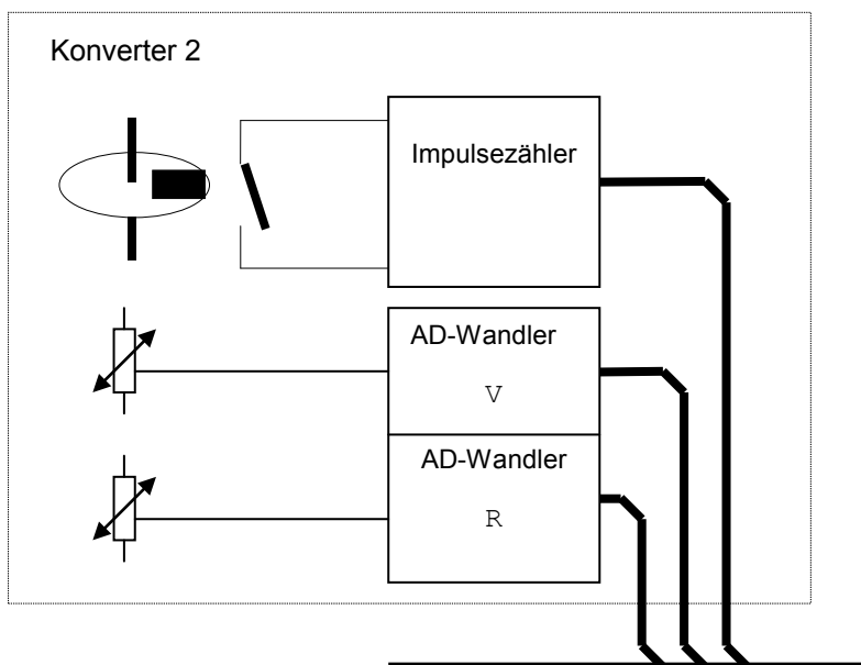
Abbildung 3: Beispiel für Messwertwandler eines Wärmehählers
