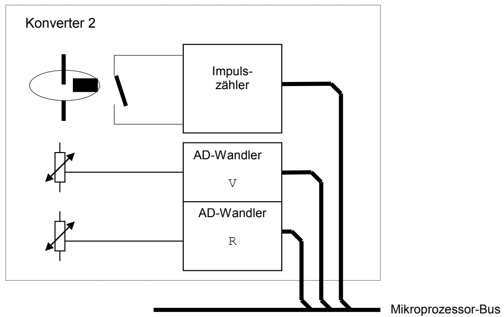
Abbildung 3: Beispiel für Messwertwandler eines Wärmehählers
