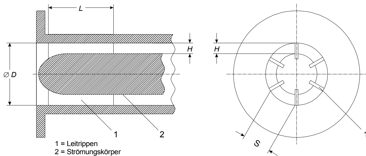
Abb.7: Maße im Einstrombereich eines axialen Turbinenradgaszählers
