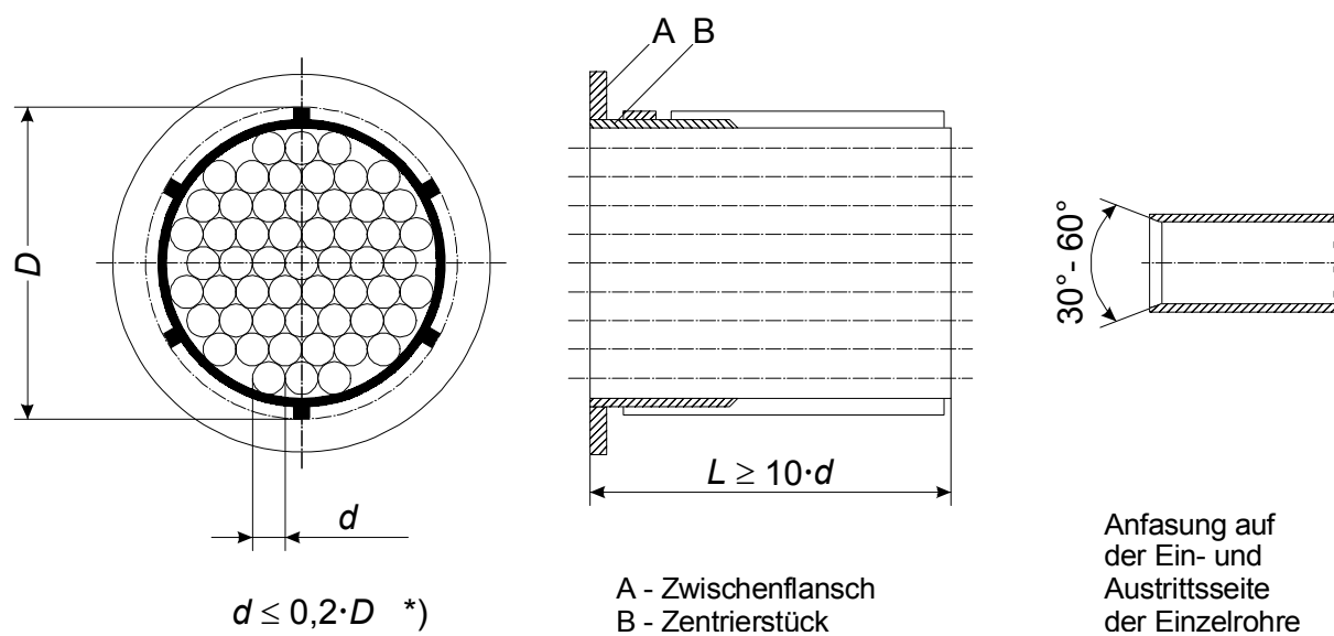
Abb.4: Rohrbündel-Gleichrichter
